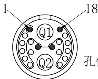
公针芯焊接端 焊接排序图
