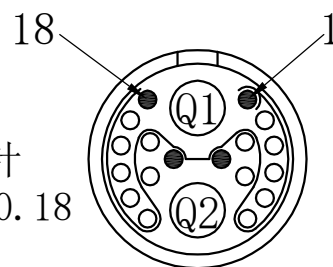
母针芯焊接端 焊接排序图
